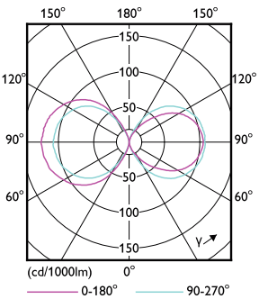
LEDTrueForce E27 360
