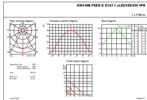
IFAS1_DN140BPSED-ED1621xLED10S830WR
