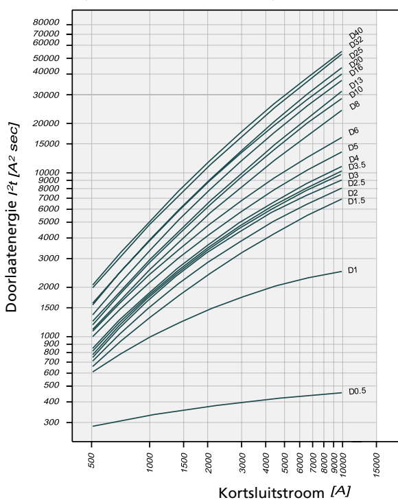
Doorlaatenergie PLSM, karakteristiek D, 1-polig
