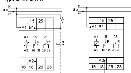
Type ZRMF2/WW
