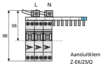
Z-SV-10/1P-F/13 Z-SV-10/N-F/13
