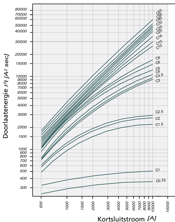
Doorlaatenergie PLSM, karakteristiek C, 1-polig
