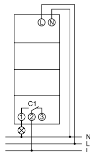
TSDW1COA
