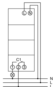
TSDW1CO
