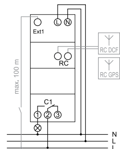
TSDW1CODG
