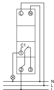
TSDW1COMIN
