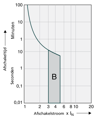
Afschakelkarakteristiek B
