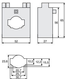
Z-MG/WAS-100 ... -400
