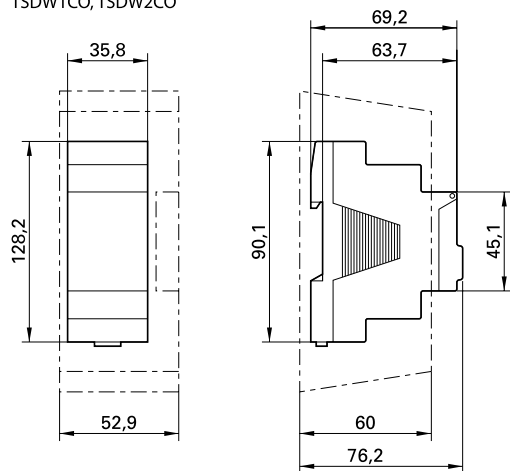
TSDW1CO, TSDW2CO
