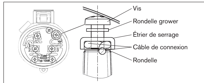
Fig. 6 : Raccordement conducteur de protection
