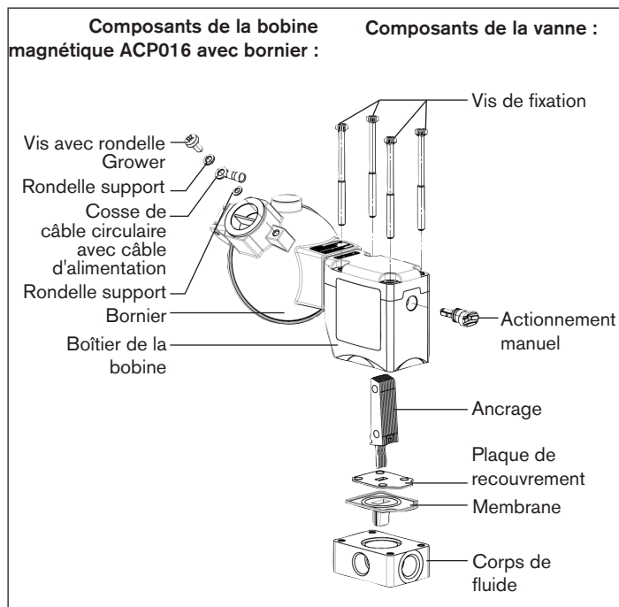
Fig. 2 : Vanne avec bobine magnétique de type ACP016 avec bornier
