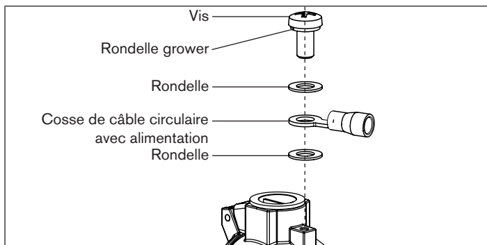
Fig. 7 : Raccordement de la compensation de potentiel externe
