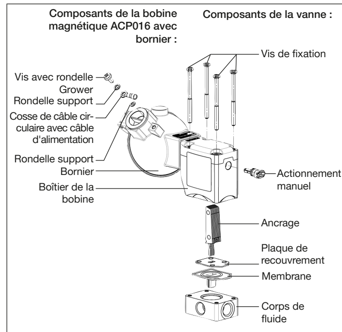
Fig. 2 : Vanne avec bobine magnétique de type ACP016 avec bornier
