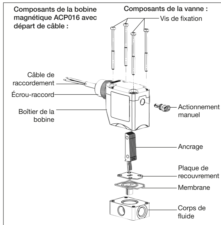
Fig. 1 : Vanne avec bobine magnétique de type ACP016 avec départ de câble
