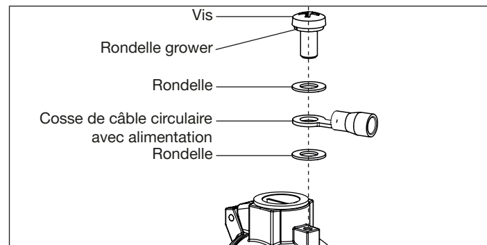
Fig. 6 : Raccordement de la compensation de potentiel externe
