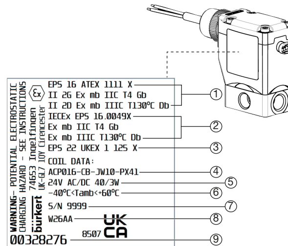
Fig. 3 : Emplacement et description de la plaque signalétique de sécurité
