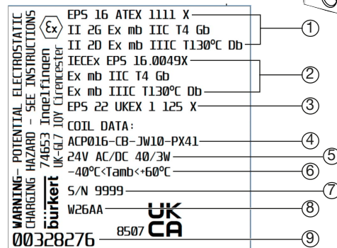
Fig. 4 : Emplacement et description des plaques signalétiques de sécurité
