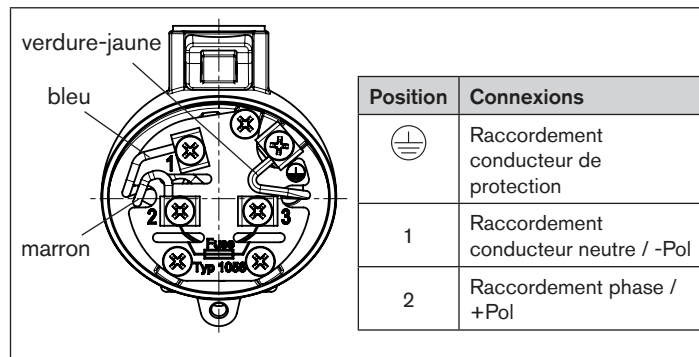
Fig. 5 : Coffret à bornes
