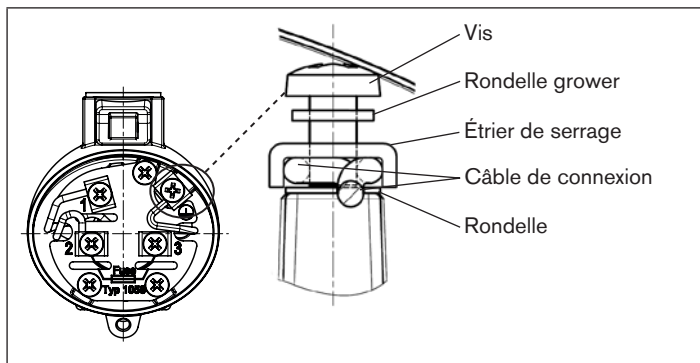
Fig. 6 : Raccordement conducteur de protection
