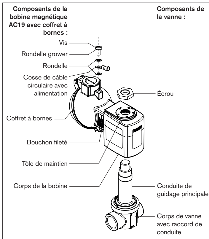
Fig. 2 : Bobine magnétique type AC19 avec coffret à bornes
