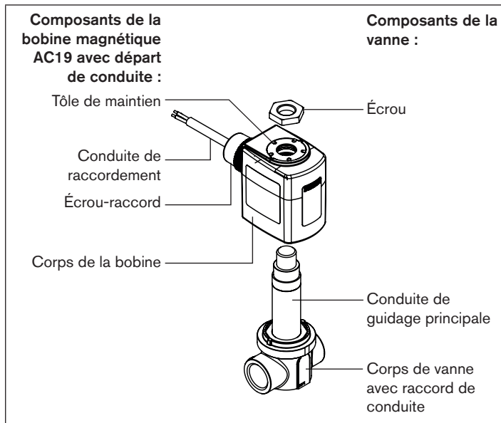
Fig. 1 : Bobine magnétique type AC19 avec départ de câble
