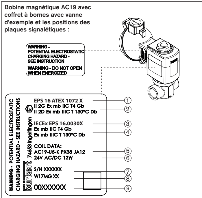
Fig. 4 : Emplacement et description des plaques signalétiques Ex
