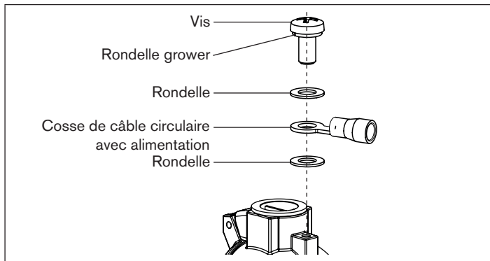
Fig. 7 : Raccordement de la compensation de potentiel externe
