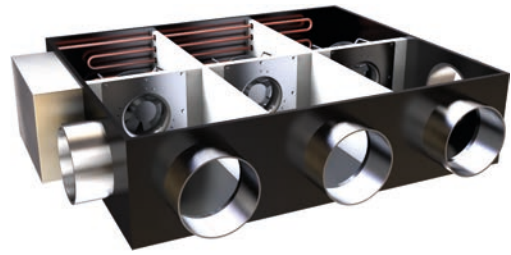
Abb. 73: Fan coil
