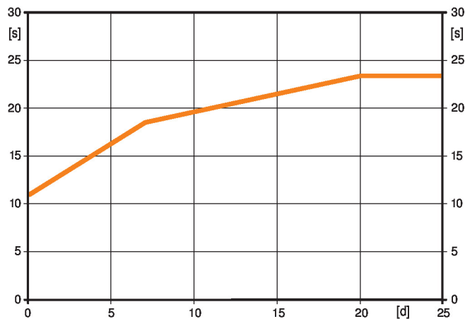
Typische Vorladezeit
