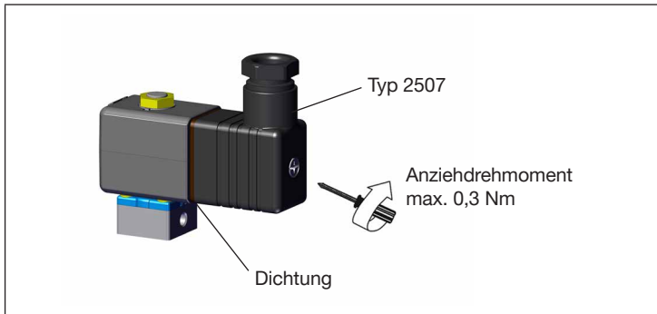
Abb. 4: Gerät elektrisch anschließen
