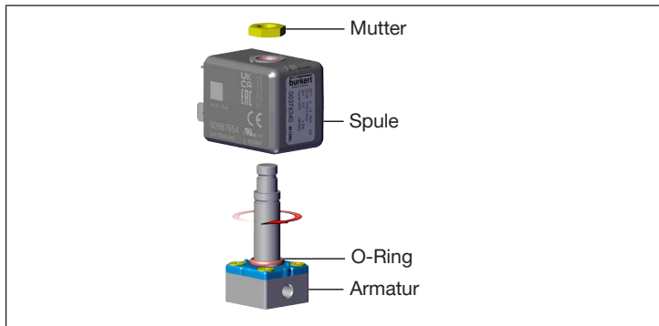
Abb. 5: Drehen der Spule
