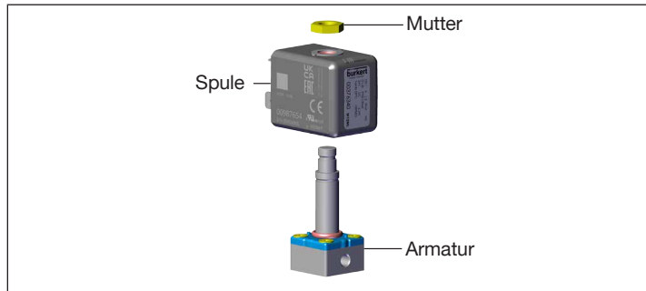
Abb. 6: Ersatzteile
